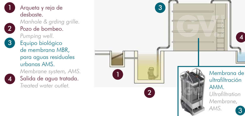
Depuradora de aguas residuales procedentes de complejos residenciales , modelo ADR. Waste water treatment from a residential complex, model ADR.
