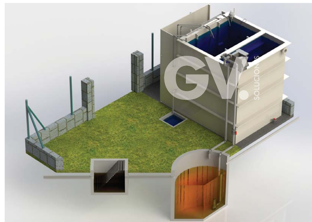
Depuradora de aguas residuales procedentes de complejos residenciales , modelo ADR. Waste water treatment from a residential complex, model ADR.
