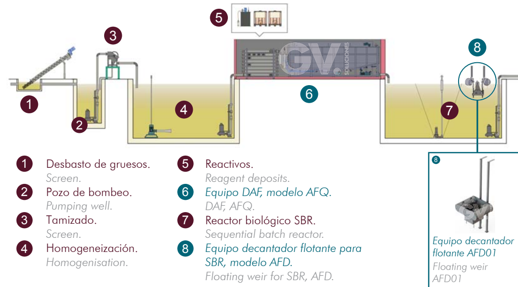
Depuradora de aguas residuales procedentes , modelo ADC. Waste water treatment for the canning industry, ADC.
