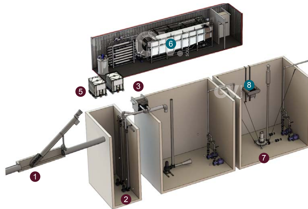
Depuradora de aguas residuales procedentes , modelo ADC. Waste water treatment for the canning industry, ADC.
