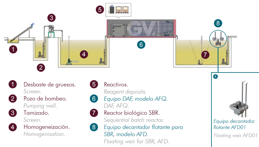
Depuradora de aguas residuales procedentes , modelo ADC. Waste water treatment for the canning industry, ADC.
