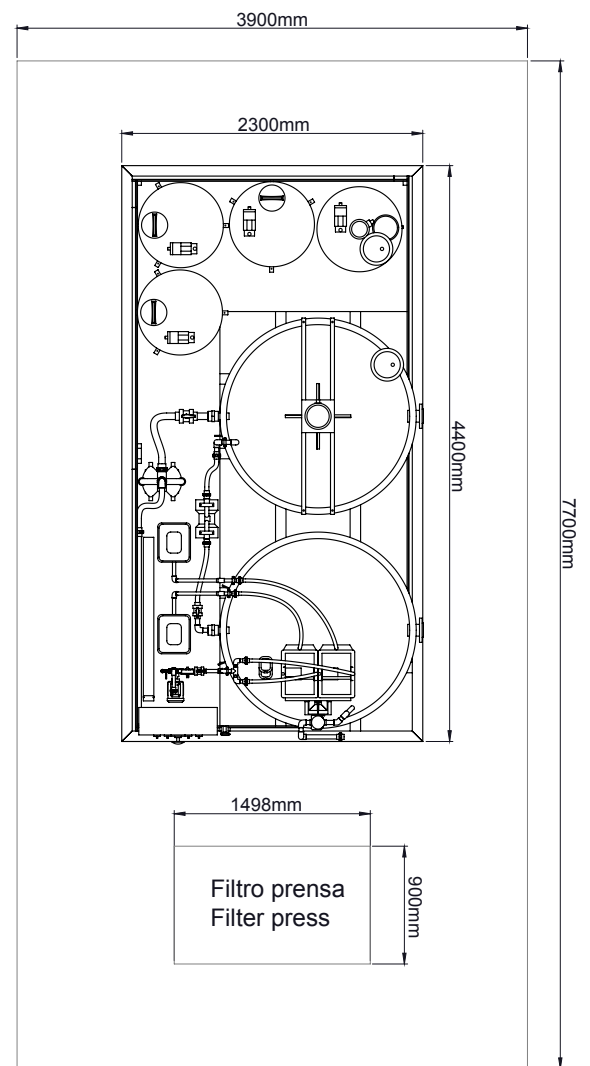
Medidas y espacio necesario para la instalación
