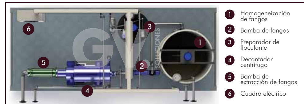
Tratamiento de fangos mediante centrifugación ASC01XXX
