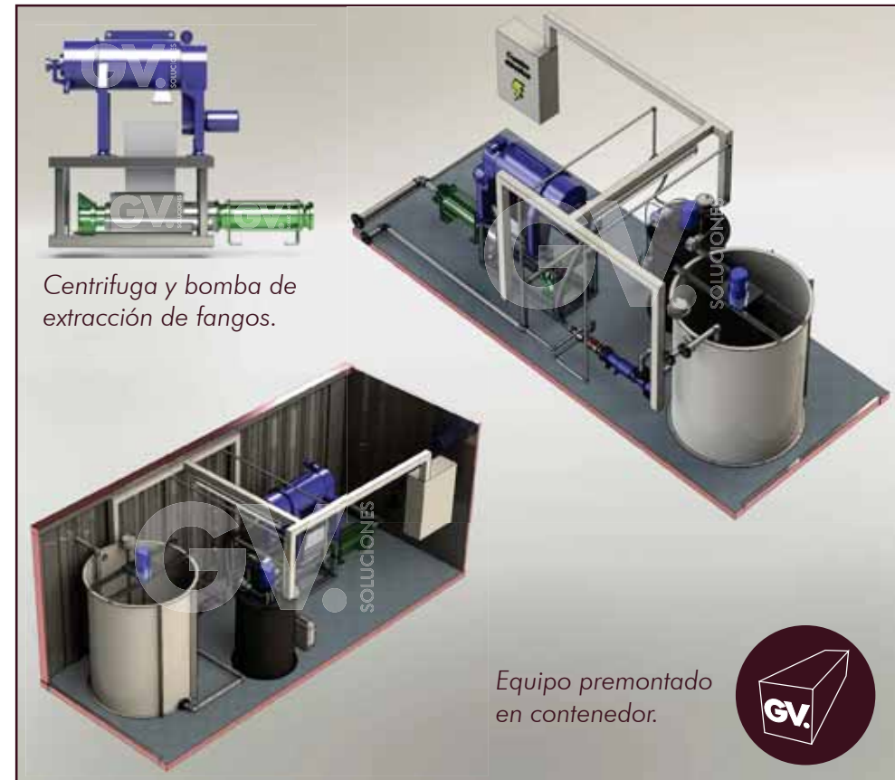
Tratamiento de fangos mediante centrifugación ASC01XXX
