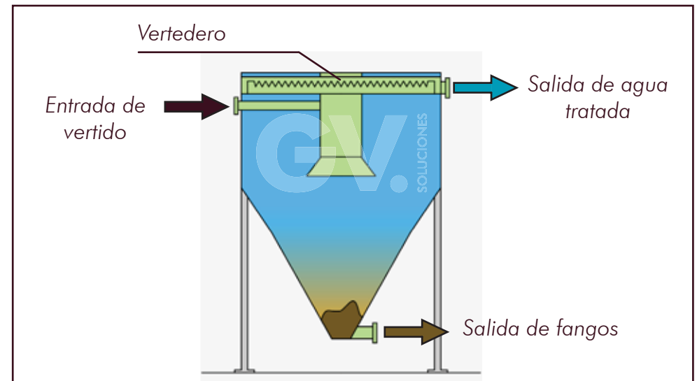
Tratamiento de fangos mediante espesadores por gravedad ASG01XXX
