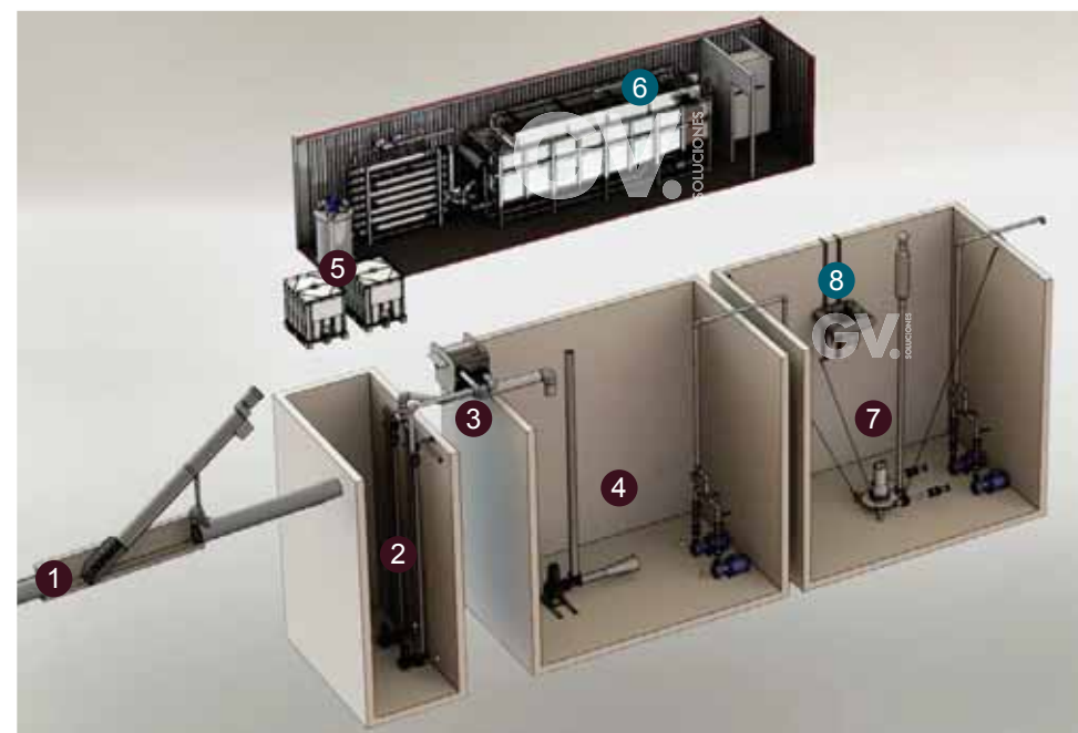
Depuradora de aguas residuales procedentes de polígonos industriales ADI01XXX.
